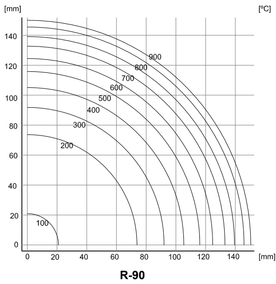
Figura C.7. Isothermas de un cuarto de sección circular de 300 mm de diámetro expuesta perimetralmente
