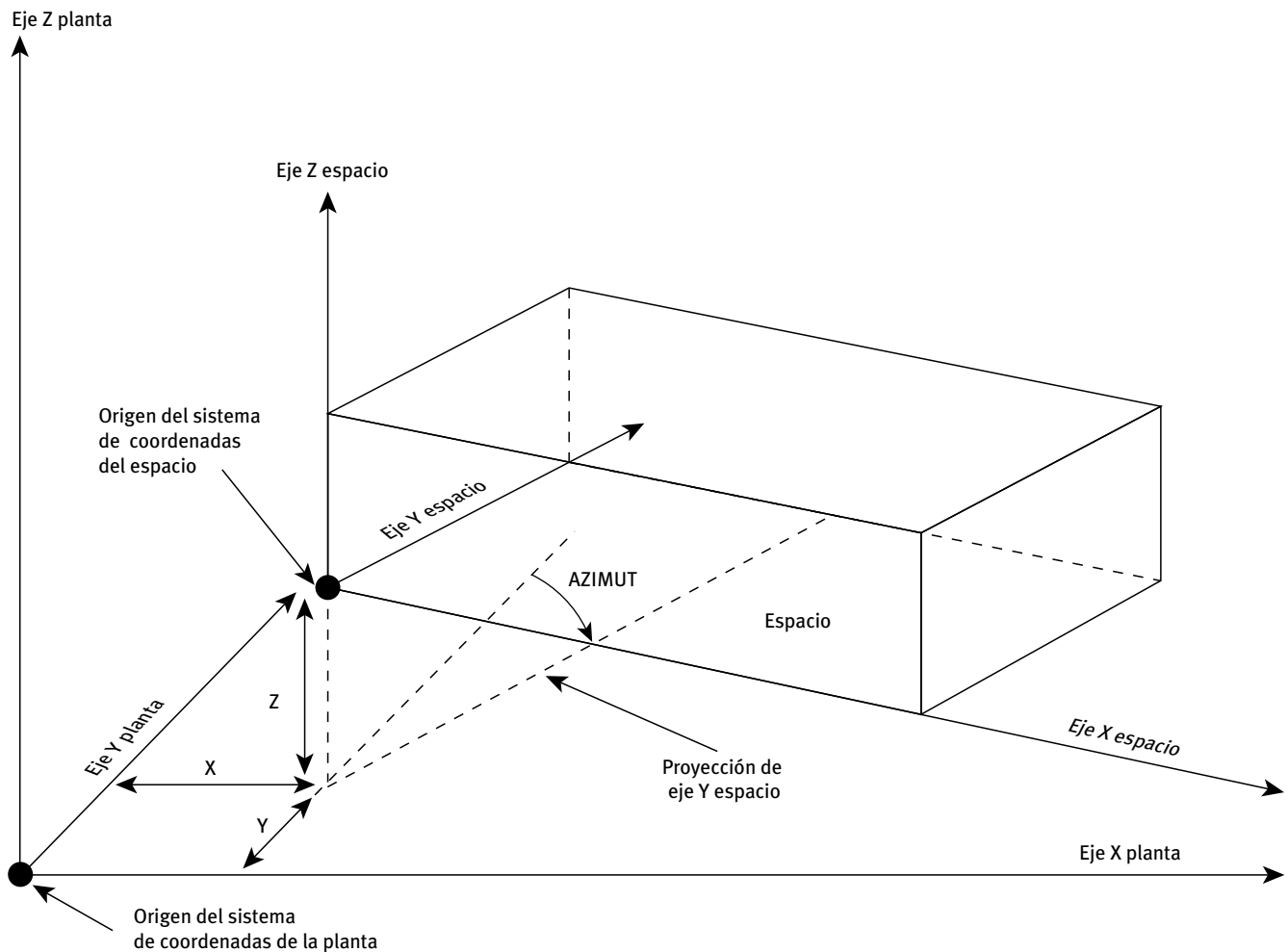
Figura 7 Localización del origen de coordenadas del objeto ESPACIO dentro del sistema de coordenadas del objeto PLANTA al cual pertenece
