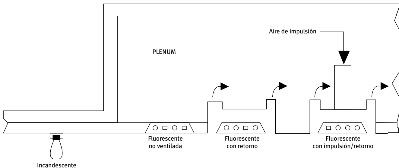
Figura 8 Esquema de los diferentes tipos de luminarias, propiedad ILUM-TIPO
