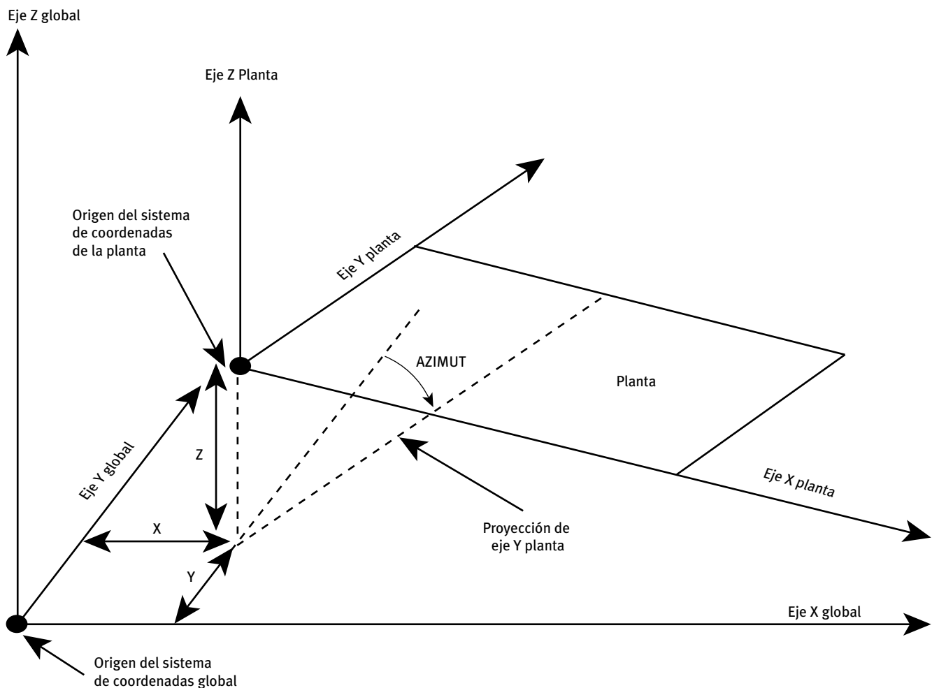
Figura 4 Localización del origen de coordenadas del objeto PLANTA dentro del sistema global de coordenadas
