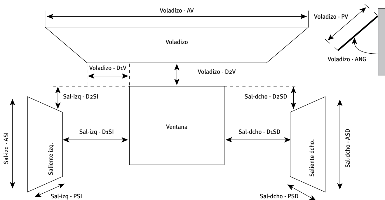
Figura 20 Propiedades para definir la geometría de los voladizos y salientes laterales en el objeto VENTANA
