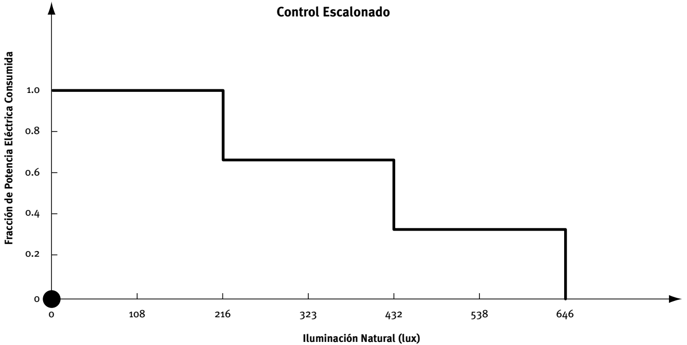
Figura 14 Ejemplo de control por etapas de iluminación, fracción de potencia eléctrica consumida
