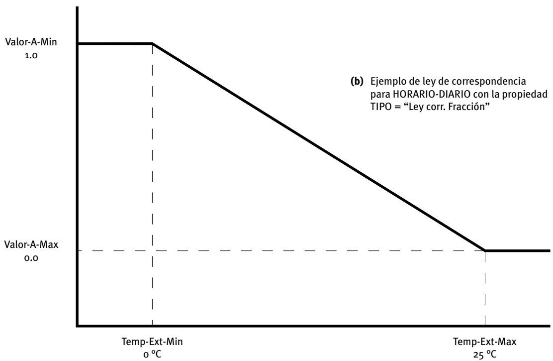
Figura 2 Ejemplo de uso de las propiedades TEMP-EXT-MAX, TEMP-EXT-MIN, VALOR-A-MAX y VALOR-A-MIN para los horarios diarios del tipo ley de correspondencia
