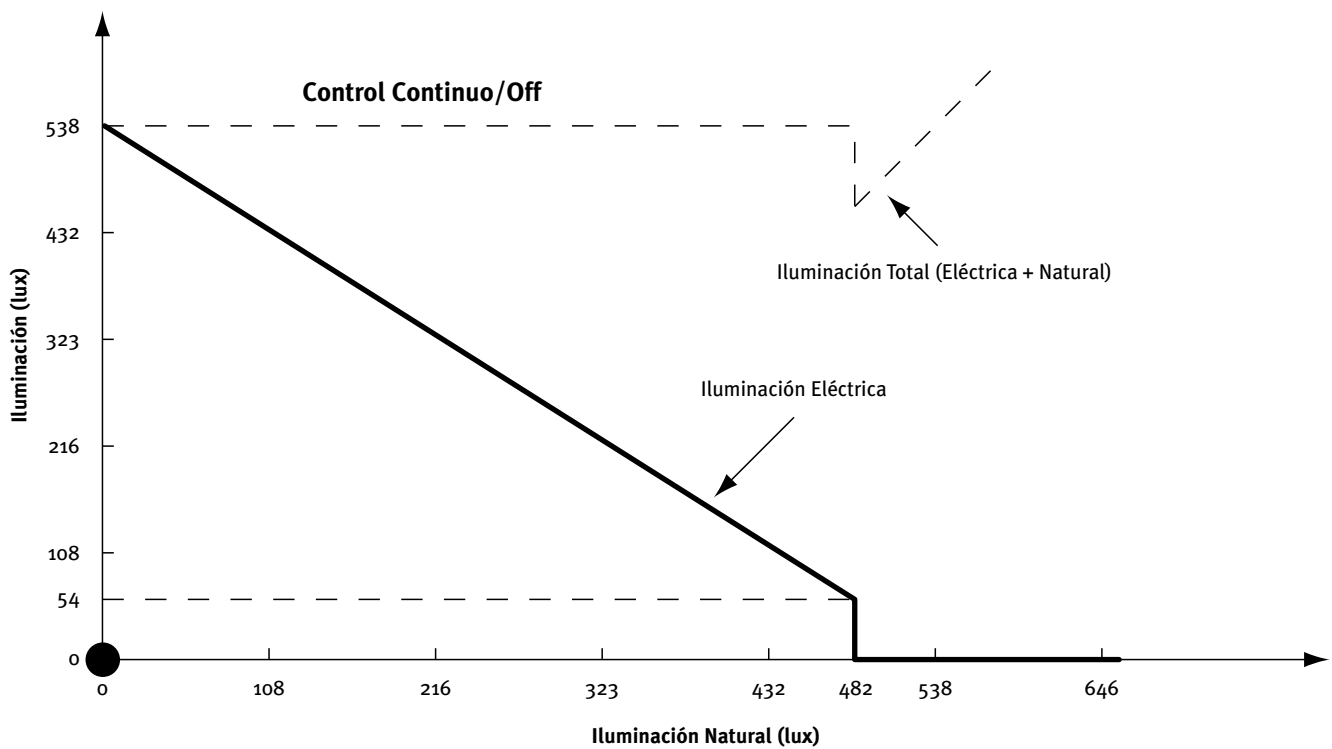
Figura 13 Ejemplo de control progresivo/apagado de iluminación, nivel de iluminación
