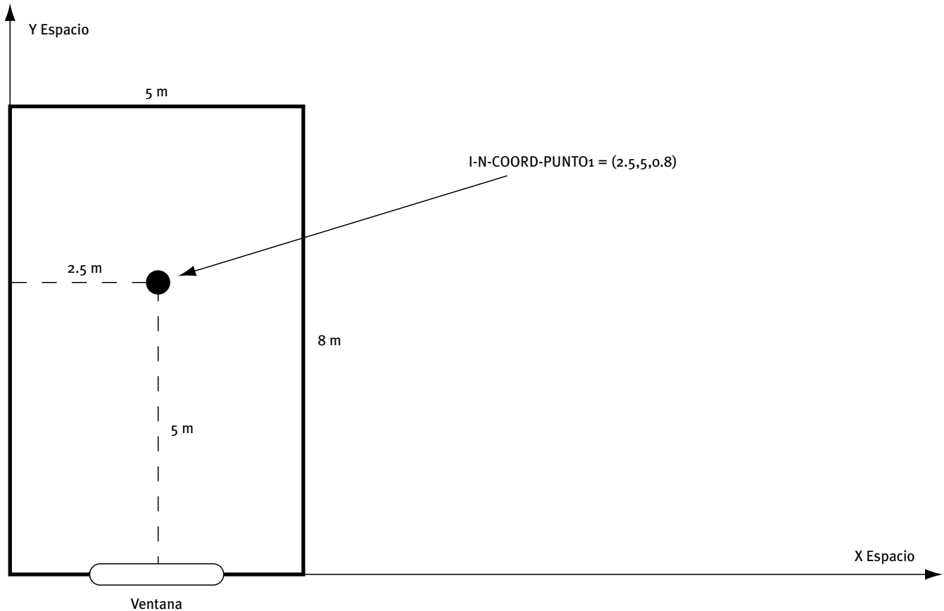
Figura 16 Ejemplo de localización mediante el uso de la propiedad I-N-COORD-PUNTO 1
