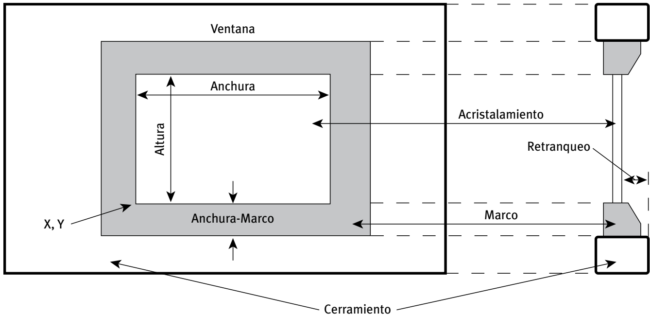
Figura 18 Propiedades geométricas principales del objeto VENTANA
