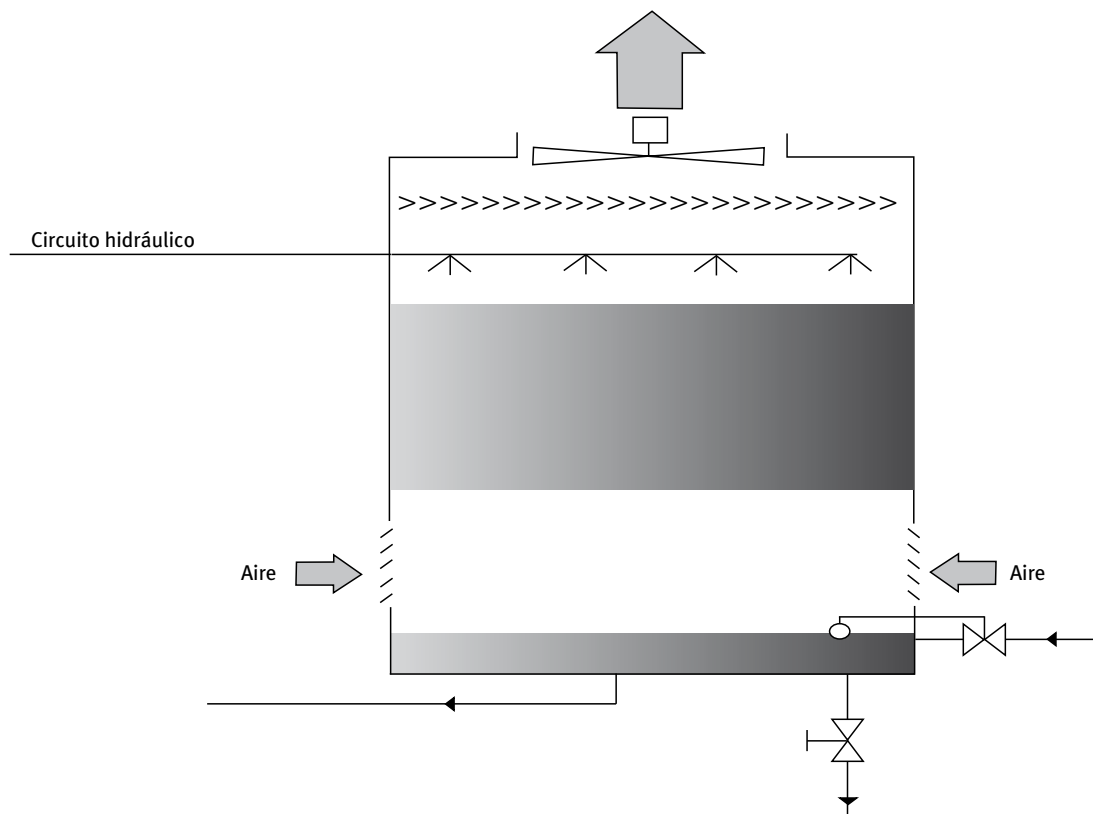
Figura 22 Esquema de torre de refrigeración con circuito abierto
