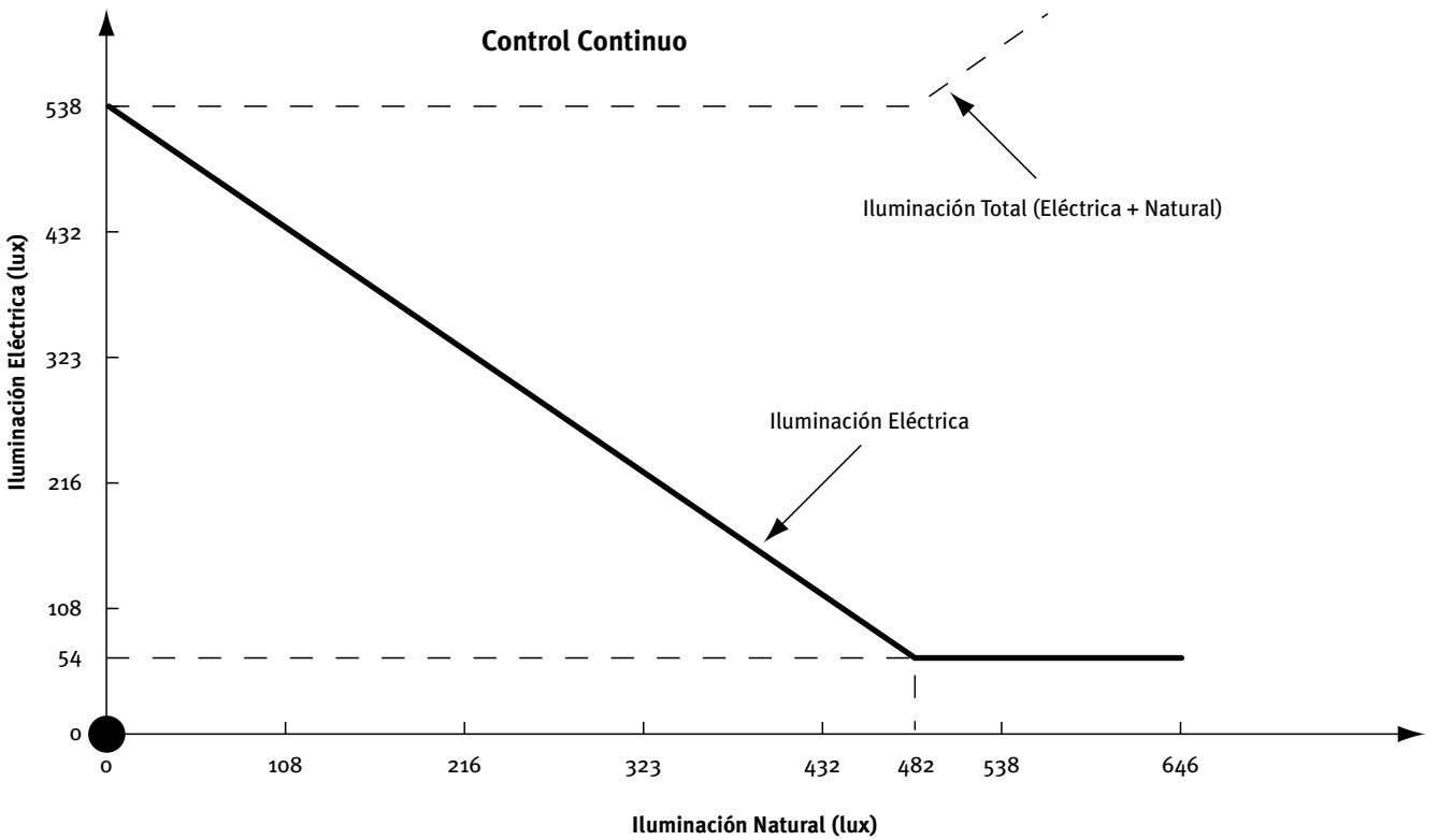
Figura 11 Ejemplo de control progresivo de iluminación, nivel de iluminación
