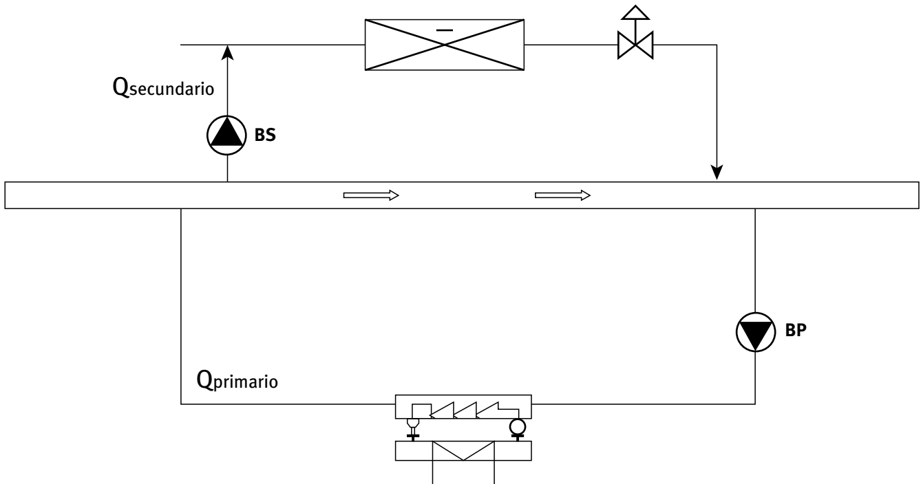
Figura 21 Recirculación de caudal de un circuito primario
