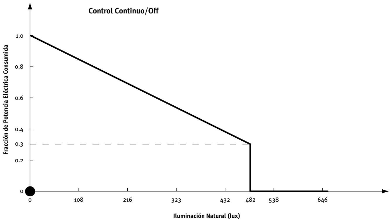
Figura 12 Ejemplo de control progresivo/apagado de iluminación, fracción de potencia eléctrica consumida
