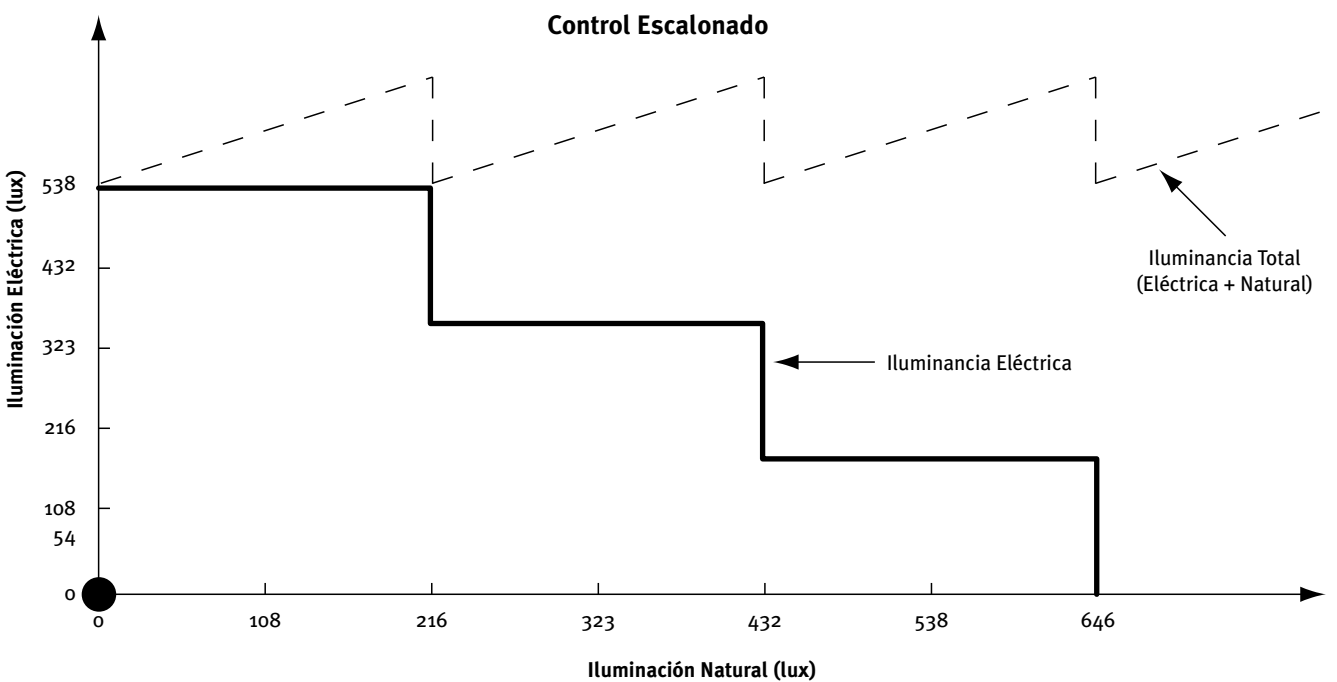
Figura 15 Ejemplo de control por etapas de iluminación, nivel de iluminación
