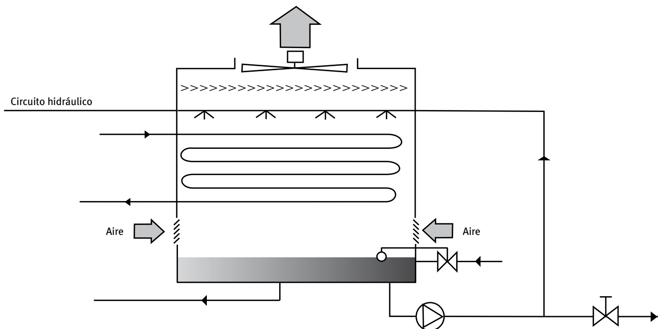
Figura 23 Esquema de torre de refrigeración con circuito cerrado
