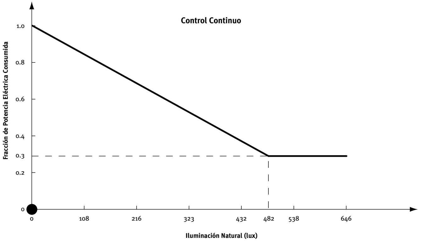
Figura 10 Ejemplo de control progresivo de iluminación, fracción de potencia eléctrica consumida
