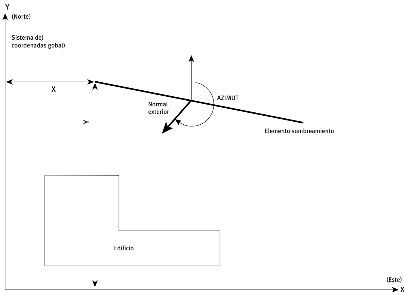
Figura 3 Localización del origen de coordenadas del objeto ELEMENTO-SOMBREAMIENTO dentro del sistema global de coordenadas
