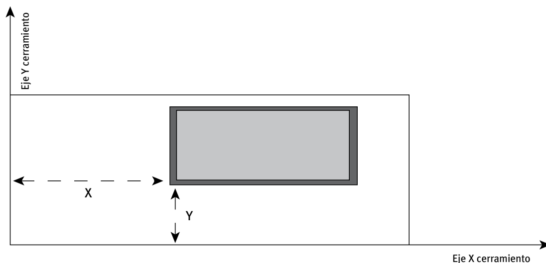
Figura 19 Localización del origen de coordenadas del objeto VENTANA dentro del sistema de coordenadas del cerramiento al cual pertenece
