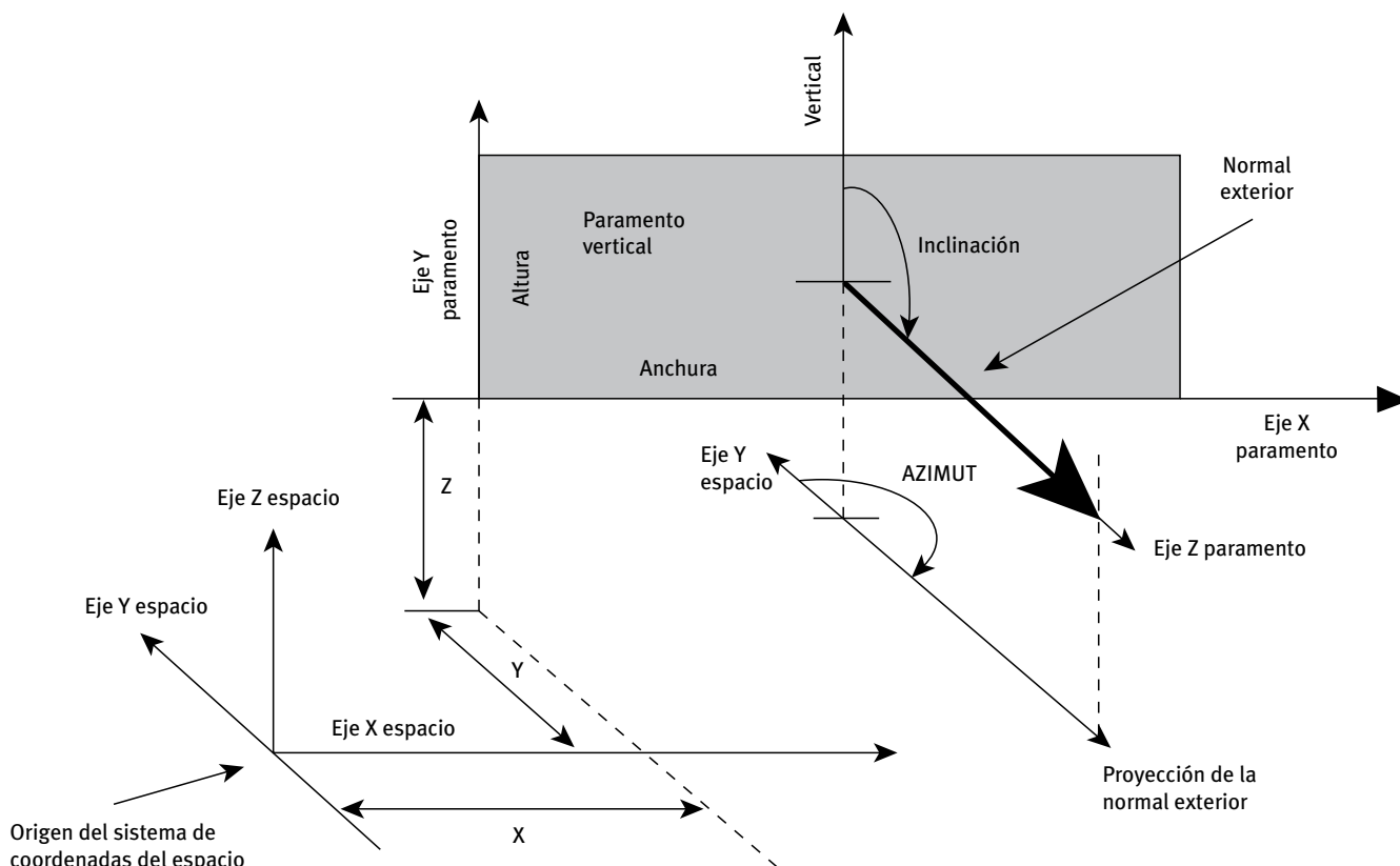
Figura 17 Localización del origen de coordenadas del objeto CERRAMIENTO-EXT dentro del sistema de coordenadas del objeto ESPACIO al cual pertenece
