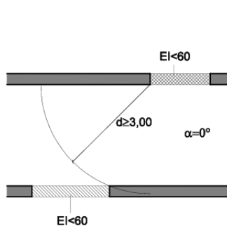
Figura 1.1. Fachadas enfrentadas
